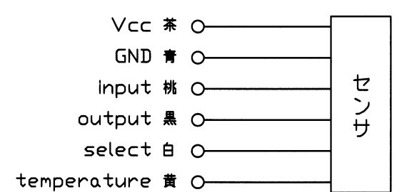
結線図
