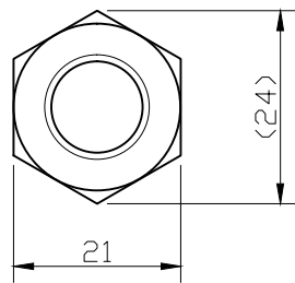
ナット形状
