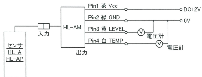
結線図
