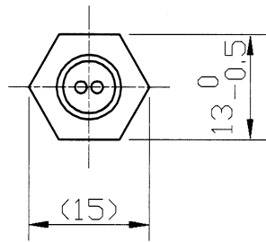
フランジ部形状
