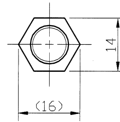
フランジ部形状
