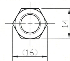
ナット形状
