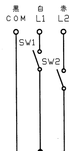
結線図
