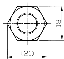
ナット形状
