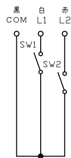
結線図
