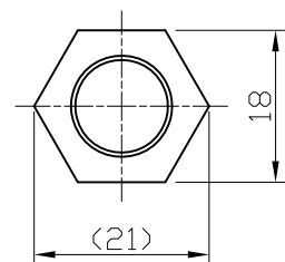
フランジ部形状
