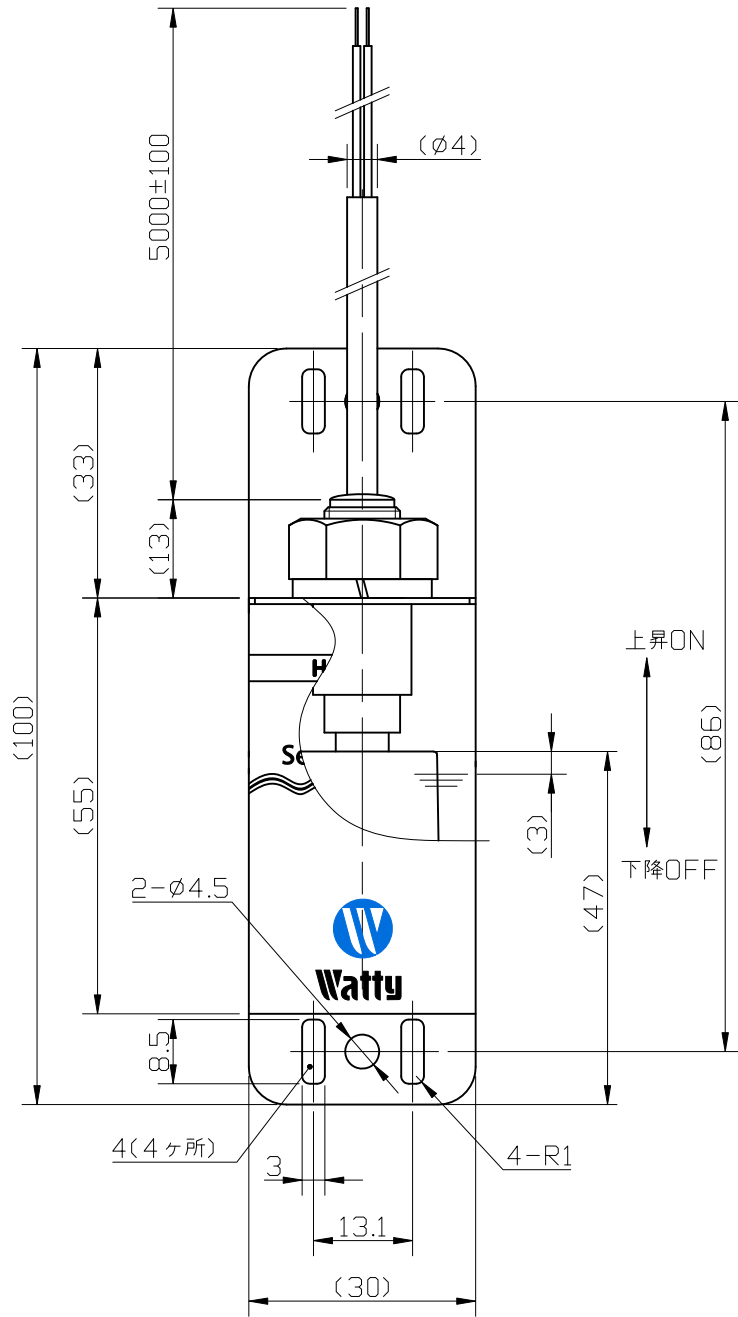
取付指示図
